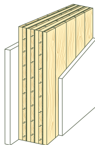
Innenwand – 7 Lagen mit beidseitiger Innen- beplankung
