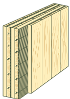
MHM-Basiswand Kreuz- und lagenweise angeordnete Bretter
