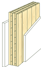
Innenwand – 5 Lagen mit beidseitiger Innen- beplankung
