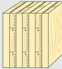
Massiv-Holz-Mauer® für warme und massive Häuser
