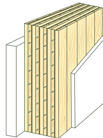
Außenwand – 9 Lagen mit Innenbeplankung und normaler Außendämmung
