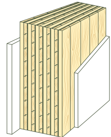
Außenwand – 11 Lagen mit Innenbeplankung und dünner Außendämmung
